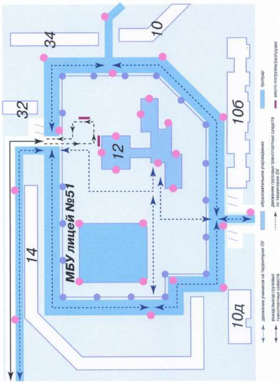
№3 СХЕМА пути движения транспортных средств к местам разгрузки/погрузки и рекомендуемые пути передвижения детей по территории МБУ лицей №51
