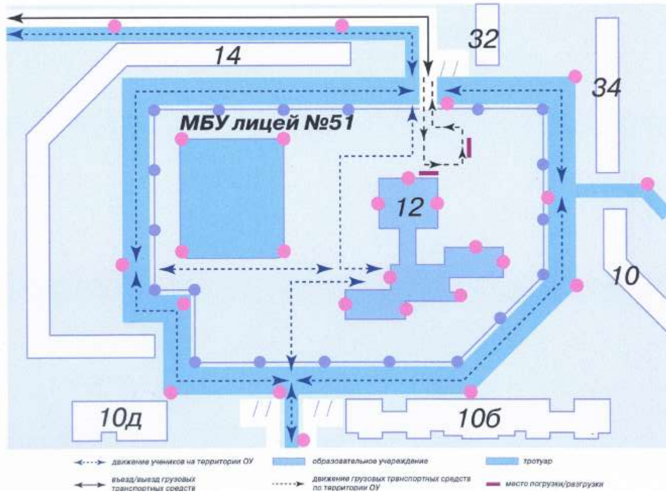
№3 СХЕМА пути движения транспортных средств к местам разгрузки/погрузки и рекомендуемые пути передвижения детей по территории МБУ лицей №51
