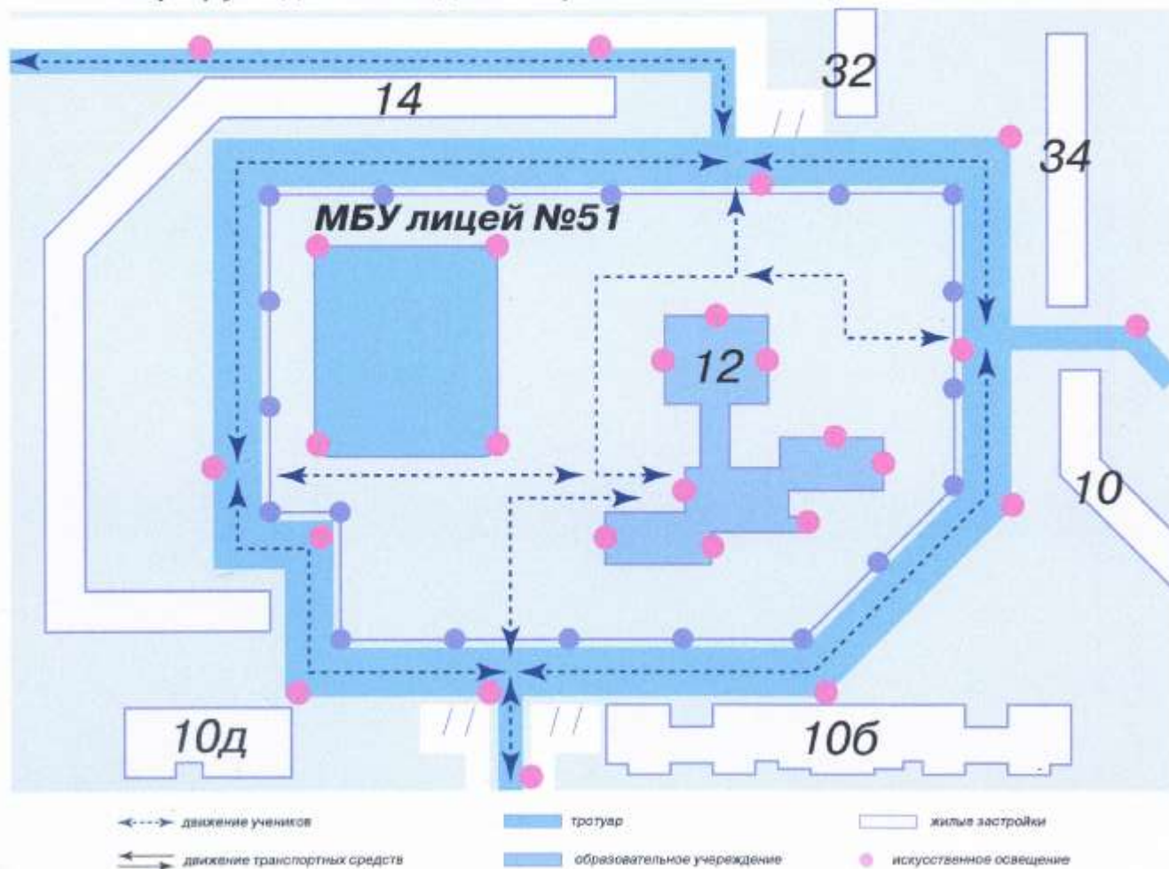
№2 СХЕМА организации дорожного движения в непосредственной близости от МБУ лицей №51, с размещением соответствующих технических средств, маршруты движения детей и расположение парковочных мест
